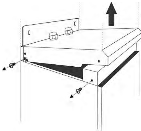
شکل ۲: نمای درپوش بالای دستگاه
